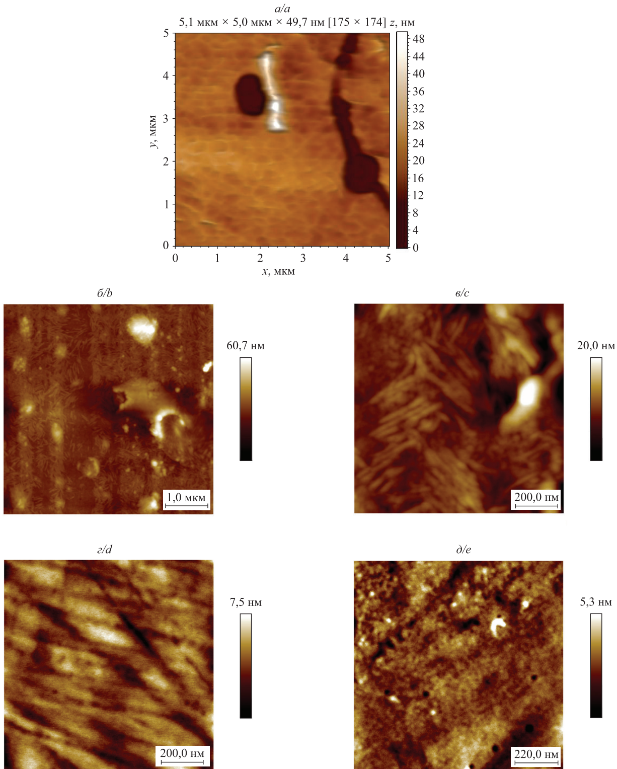
Рис. 1. Структура пленок ПММА, сформированных на обезжиренных кремниевых пластинах ( a , d ) и предметных стеклах ( b , c , e ) из раствора с концентрацией 1 мг/мл методами полива ( a – b ) и спин-коутинга ( d , e ) Fig. 1. The structure of PMMA films formed on the degreased surface of silicon wafers ( a , d ) and glass slides ( b , c , e ) from solution with a concentration 1 mg/mL by watering ( a – c ) and spin-coating ( d , e ) methods
