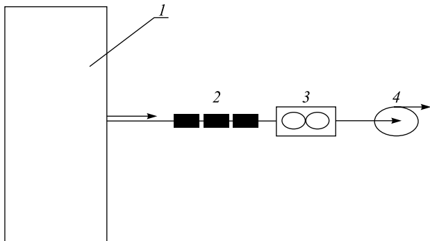
Рис. 1. Схема устройства для извлечения ПАУ из отходящих газов: 1 – пиролизная установка; 2 – три последовательно соединенных картриджа; 3 – расходомер; 4 – насос
