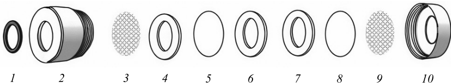
Рис. 2. Устройство разъемного картриджа: 1 – уплотнительное кольцо; 2 и 10 – корпус картриджа; 3 и 9 – металлическая сетка; 4, 6 и 7 – кольцо для закрепления фильтра; 5 и 8 – стекловолоконные фильтры, между которыми засыпается твердый адсорбент Supelpak-2
