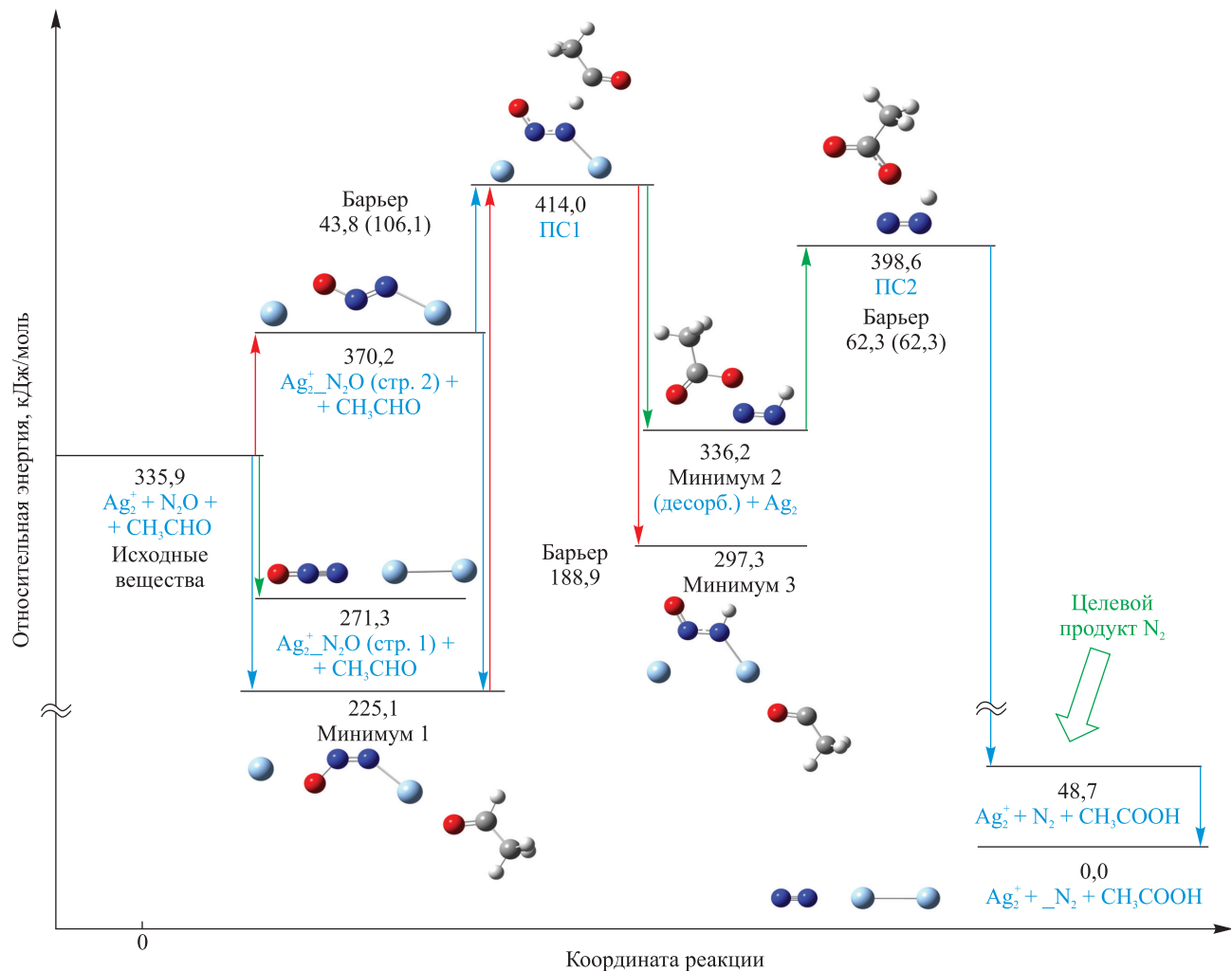
Рис. 4. Энергетическая диаграмма реакции восстановления \text{N}_2\text{O} до \text{N}_2 в случае катализаторов с высоким содержанием серебра на примере каталитических центров \text{Ag}_2^+ . В скобках указаны величины барьеров аналогичных процессов на каталитических центрах \text{Ag}_2 .
