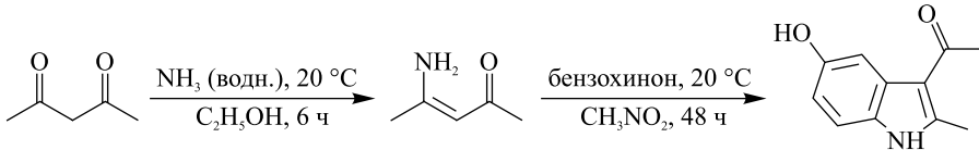
Рис. 1. Схема синтеза 5-НІЕТ
