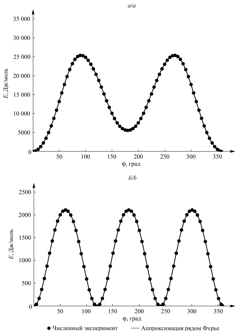
Рис. 2. Потенциальные функции вращения в молекуле темозоломида: a – амидный волчок; b – метильный волчок
