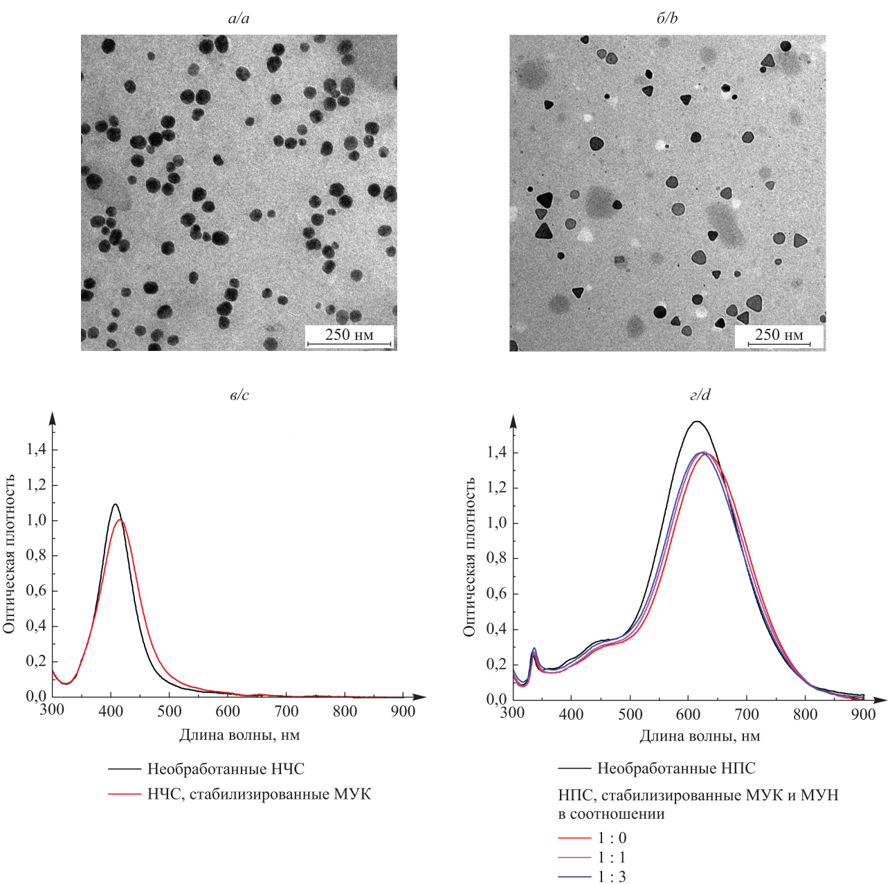
Рис. 1. ПЭМ-снимки индивидуальных квазисферических НЧС ( а ) и НПС ( б ), спектры экстинкции водных коллоидных растворов квазисферических НЧС ( в ) и НПС ( г ) до и после обработки МУК либо смесями МУК и МУН
