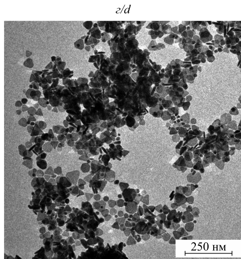
Рис. 3. ПЭМ-снимки НПС и их агрегатов до смешения с буферами (а) и спустя 3 ч после смешения с Li-фосфатным (б), Na-фосфатным (в) и Cs-фосфатным (г) буферами с pH 8,0 и концентрацией 0,02 моль/л
