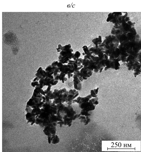
Рис. 3. ПЭМ-снимки НПС и их агрегатов до смешения с буферами (а) и спустя 3 ч после смешения с Li-фосфатным (б), Na-фосфатным (в) и Cs-фосфатным (г) буферами с pH 8,0 и концентрацией 0,02 моль/л
