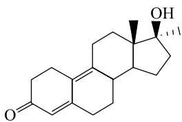
Метилдиенолон (MDNL)
