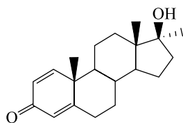
Метандиенон (MTDE)
