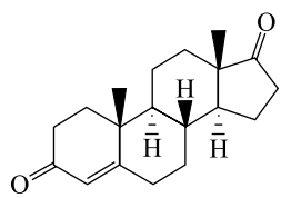
4-Андростен-3,17-дион (ADON)
