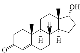
Эпитестостерон (EpiTesto)
