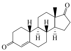
19-Норандростендион (NADON)
