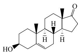
Дегидроэпиандростерон (DHEA)
