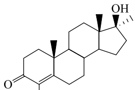
Клостебол (CLSB)
