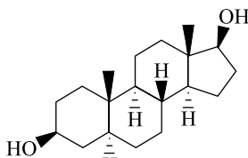
5α-Андростан-3β,17β-диол (3b-diol)
