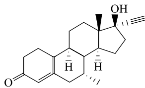
Тиболон (Tibn)
