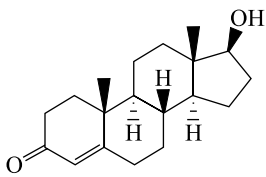
Тестостерон (Testo)
