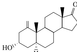
1-Метил-5α-андростан-3α-ол-17-он (METN-M1)
