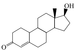
Нандролон (NAND)
