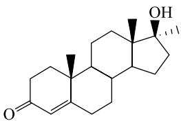
17α-Метилтестостерон (MTSN)
