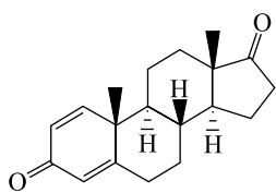
1,4-Андростадиен-3,17-дион (BOLDIONE)
