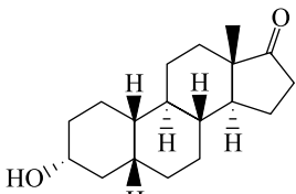
19-Норэтиохоланолон (NETC)
