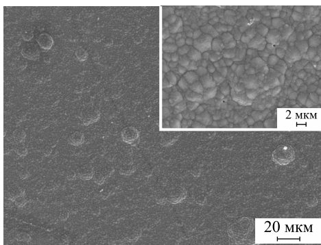
Рис. 2. СЭМ-фотографии поверхности покрытий Ni – Sn толщиной 1 мкм ( а, в ), 5 мкм ( б, г ) и 10 мкм ( д ), осаждаемых из ЭГ электролитов № 4 ( а, б ) и № 5 ( в – д ) при плотности тока 0,5 А/дм 2
