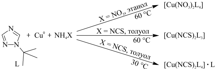
Рис. 2. Схема прямого синтеза КС 1- tert -бутил-1 H -1,2,4-триазола
