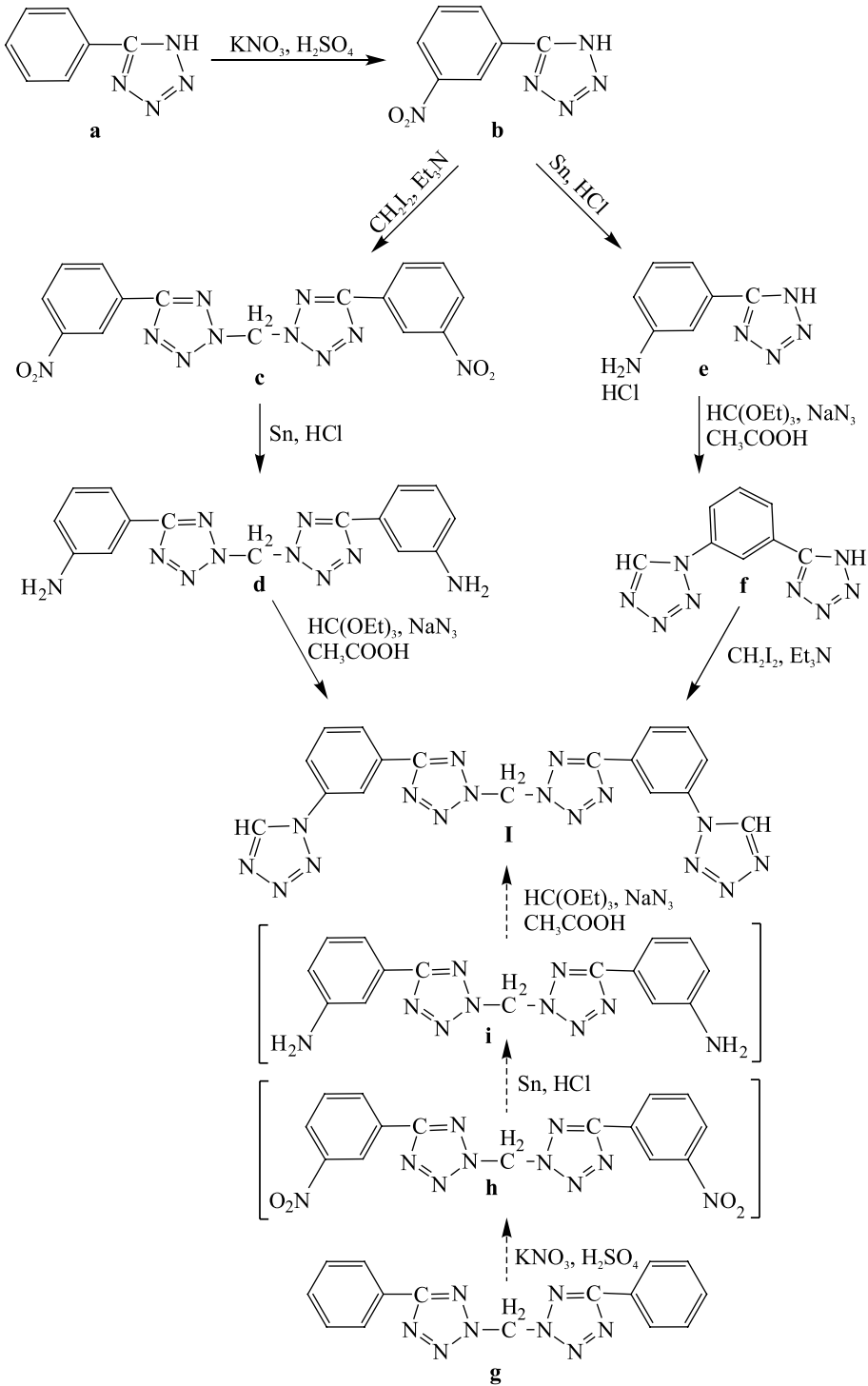
Рис. 1. Схема синтеза бис(5-(3-(тетразол-1-ил)фенил)тетразол-2-ил)метана (I): a → b → c → d (метод А), a → b → e → f (метод В), g → h → i (метод С)
