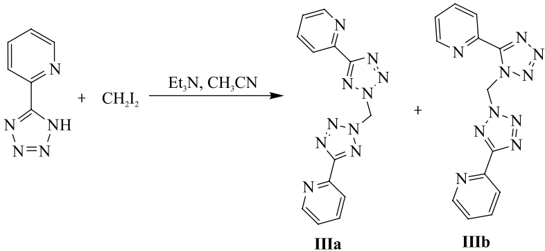
Рис. 3. Схема алкилирования 2-(тетразол-5-ил)пиридина диодометаном
