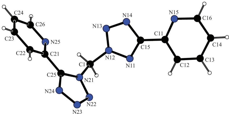
Рис. 4. Структура молекулы (5-(пиридин-2-ил)тетразол-2-ил)(5-(пиридин-2-ил)тетразол-1-ил)метана ( IIIb )
