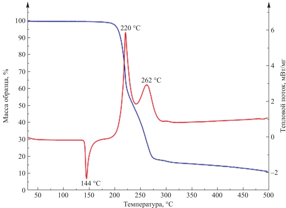
Рис. 2. Графики ТГА и ДСК для соединения 2
