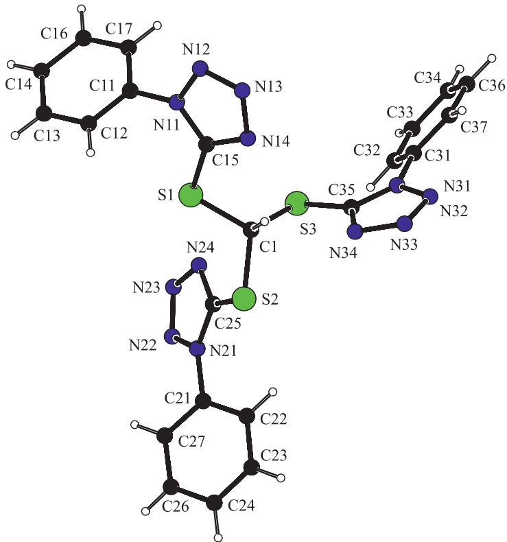
Рис. 5. Структура молекулы соединения 3a с нумерацией неводородных атомов
