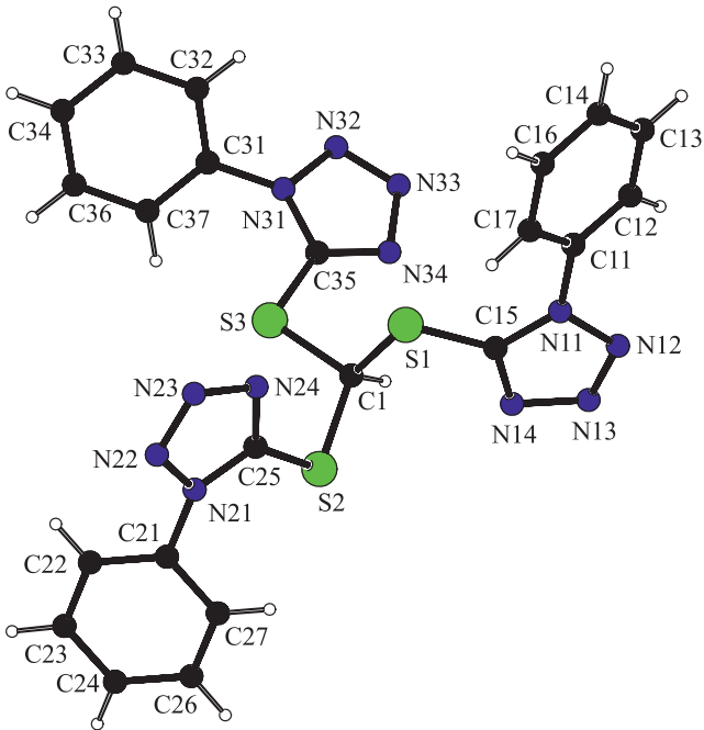
Рис. 6. Структура молекулы соединения 3b с нумерацией неводородных атомов
