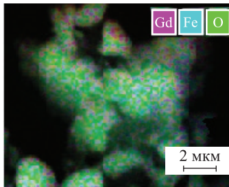
Рис. 1. Изображение СЭМ (а) и картирование элементного состава (б) порошка \text{Fe}_{2.9}\text{Gd}_{0.1}\text{O}_4 Fig. 1. SEM image (a) and elemental composition mapping (b) of \text{Fe}_{2.9}\text{Gd}_{0.1}\text{O}_4 powder
