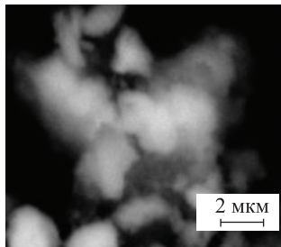
Рис. 1. Изображение СЭМ (а) и картирование элементного состава (б) порошка \text{Fe}_{2.9}\text{Gd}_{0.1}\text{O}_4 Fig. 1. SEM image (a) and elemental composition mapping (b) of \text{Fe}_{2.9}\text{Gd}_{0.1}\text{O}_4 powder
