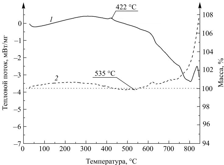
Рис. 2. Кривые дифференциальной сканирующей калориметрии (1) и термогравиметрии (2), полученные для покрытия никель – бор, осажденного из электролита, содержащего 0,1 г/л морфолин-борана
