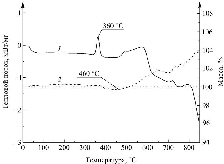
Рис. 5. Кривые дифференциальной сканирующей калориметрии (1) и термогравиметрии (2), полученные для покрытия никель – бор, осажденного из электролита, содержащего 0,4 г/л декагидро-κлозо-декабората натрия
