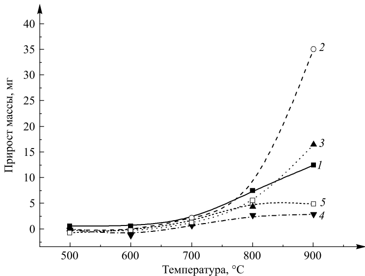
Рис. 6. Зависимость прироста массы никелевого покрытия (1) и покрытий никель – бор, осажденных из электролита, содержащего 0,1 г/л (2) и 0,4 г/л (3) морфолин-борана, 0,1 г/л (4) и 0,4 г/л (5) декагидро-клозо-декабората натрия, от температуры прогрева (продолжительность прогрева 6 ч)
