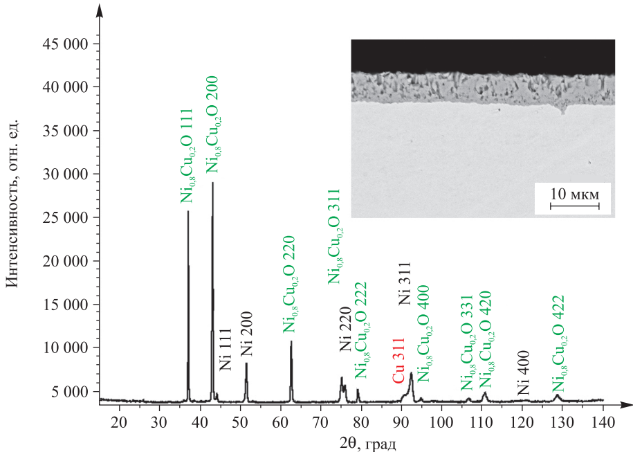
Рис. 8. Фрагмент дифрактограммы никелевого покрытия после прогрева при 800 °С. СЭМ-изображение поперечного шлифа покрытия (вставка)
