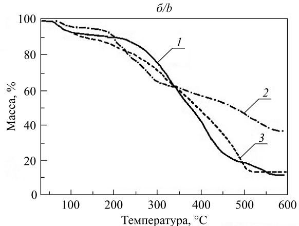
Рис. 7. Данные ТГ для образцов древесины (а) и торфа (б): 1 – индивидуальный образец; 2 – образец, обработанный ОС-4; 3 – образец, обработанный ОС-2
