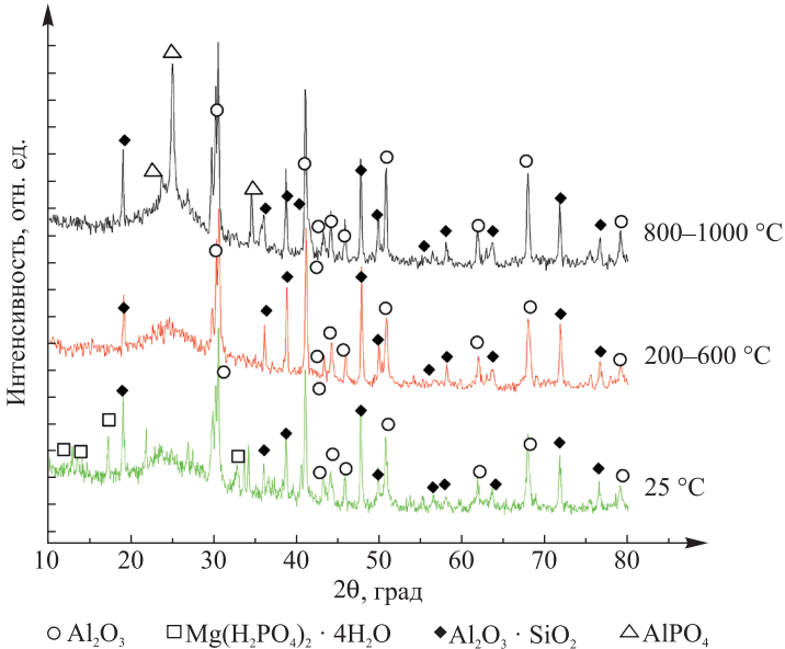
Рис. 6. Рентгенограммы образцов термостойкого магний-фосфатного композита с зольными ПМС, обработанных при различных температурах
