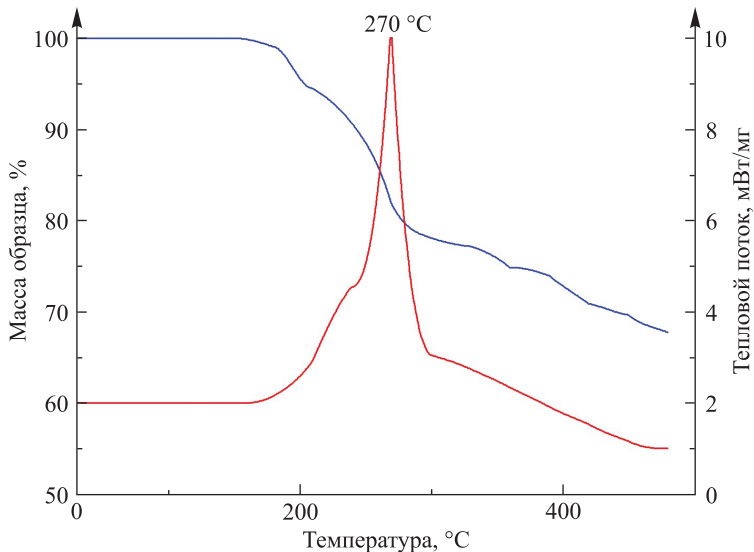
Рис. 2. Кривые термогравиметрического анализа и дифференциальной сканирующей калориметрии, полученные для 3,6-ди(тетразол-1-ил)карбазола Fig. 2. Thermogravimetric analysis and differential scanning calorimetry plots for 3,6-di(tetrazol-1-yl)carbazole
