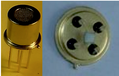
Рис. 2. Фотографические снимки сенсора (а) и чувствительных элементов на основе \text{SnO}_2 (б) и \text{In}_2\text{O}_3 (в)
