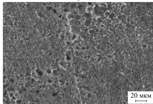
Рис. 2. СЭМ-изображения образцов магниевого сплава МА2-1 после обработки в растворе, содержащем 120 г/л \text{CrO}_3 и 110 мл/л (63 %) \text{HNO}_3 .
