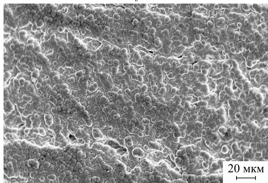
Рис. 6. СЭМ-изображения образцов магниевого сплава МА2-1 после осаждения покрытия никель – фосфор с предварительным травлением в растворе, содержащем 120 г/л \text{CrO}_3 , 110 мл/л (63 %) \text{HNO}_3 , продолжительностью 10 с (а), 20 с (б), 30 с (в), 40 с (г), 50 с (д), 60 с (е)
