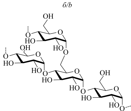
Рис. 1. Структурные формулы амилозы ( a ) и амилопектина ( б ) крахмала
