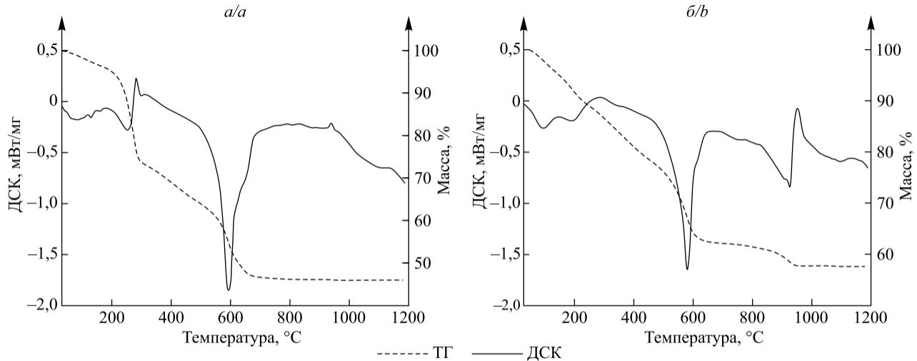
Рис. 1. Кривые ТГ и ДСК для аммиачного (а, образец 3) и карбонатного (б, образец 1) прекурсоров Fig. 1. Thermogravimetric and differential scanning calorimetry curves for ammonia (a, sample 3) and carbonate (b, sample 1) precursors
