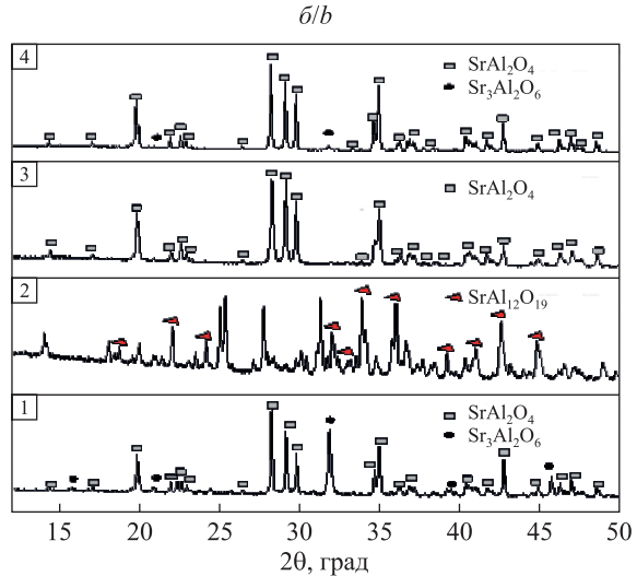
Рис. 3. Рентгенограммы образцов 1, 2, 3, 4, прогретых при 1200 °С (а) и 1500 °С (б)
