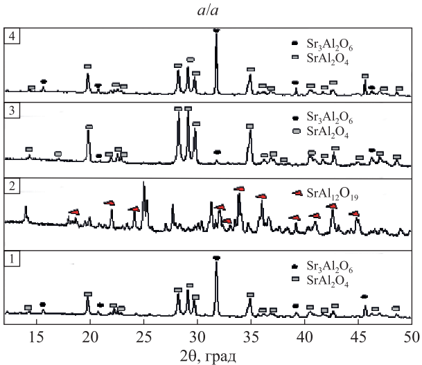
Рис. 3. Рентгенограммы образцов 1, 2, 3, 4, прогретых при 1200 °С (а) и 1500 °С (б)
