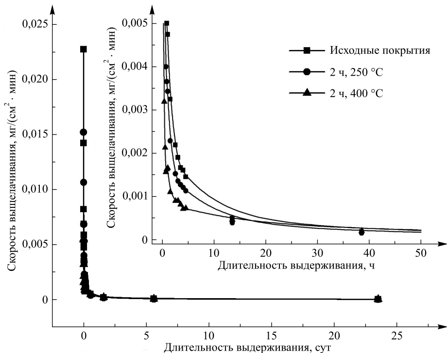
Рис. 4. Зависимость скорости выщелачивания покрытий от длительности выдерживания в 7,5 \text{ моль}/\text{дм}^3 растворе NaOH при комнатной температуре до и после прогрева при 250 и 400 °C
