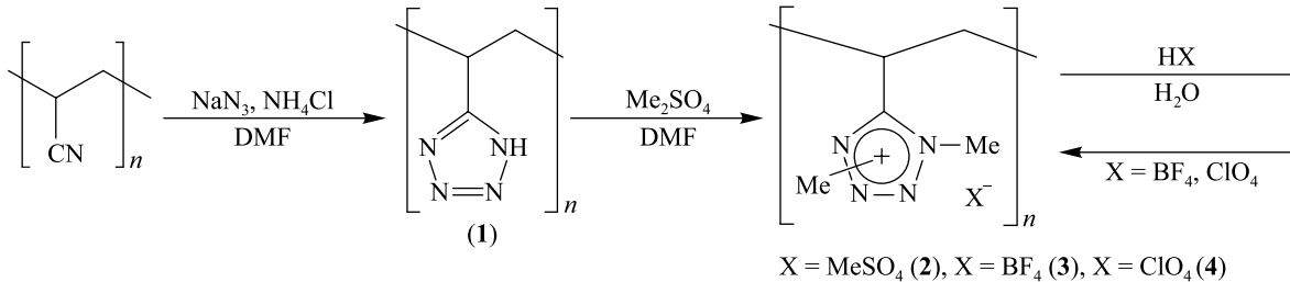
Рис. 1. Схема синтеза солей поли-5-винил-N,N'-диметилтетразолия
