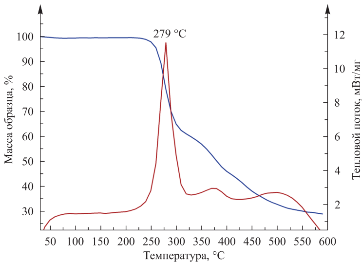
Рис. 2. Графики ТГА и ДСК для полимера (4)
