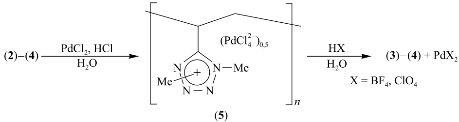
Рис. 3. Химическая схема процессов сорбции и десорбции Pd(II) солями поли-5-винил-N,N'-диметилтетразолия
