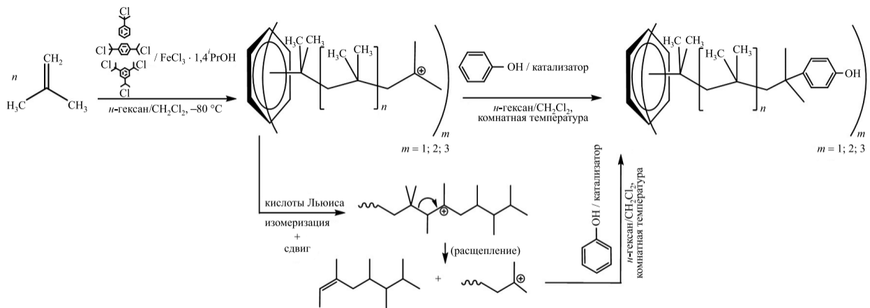
Рис. 2. Схема синтеза ПИБ-ОН различной функциональности без стадии выделения полимера Fig. 2. Scheme of PIB-OH synthesis with different functionalities without the polymer isolation
