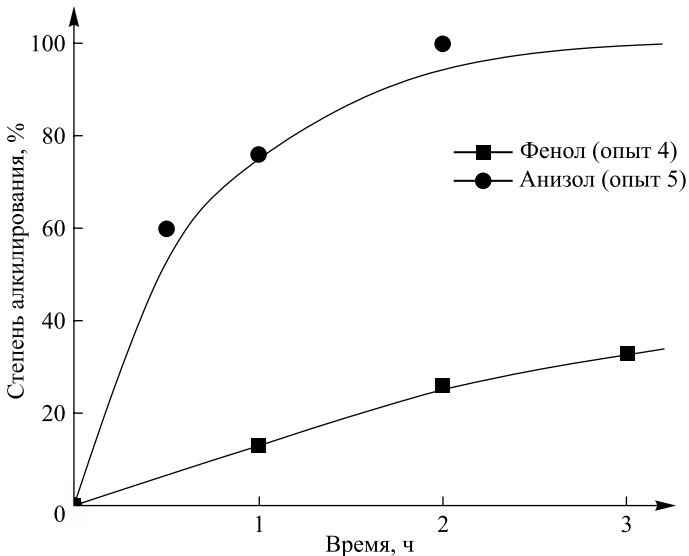
Рис. 3. Зависимость степени алкилирования субстрата ПИБ от времени для опытов 4 и 5 (см. табл. 1)
