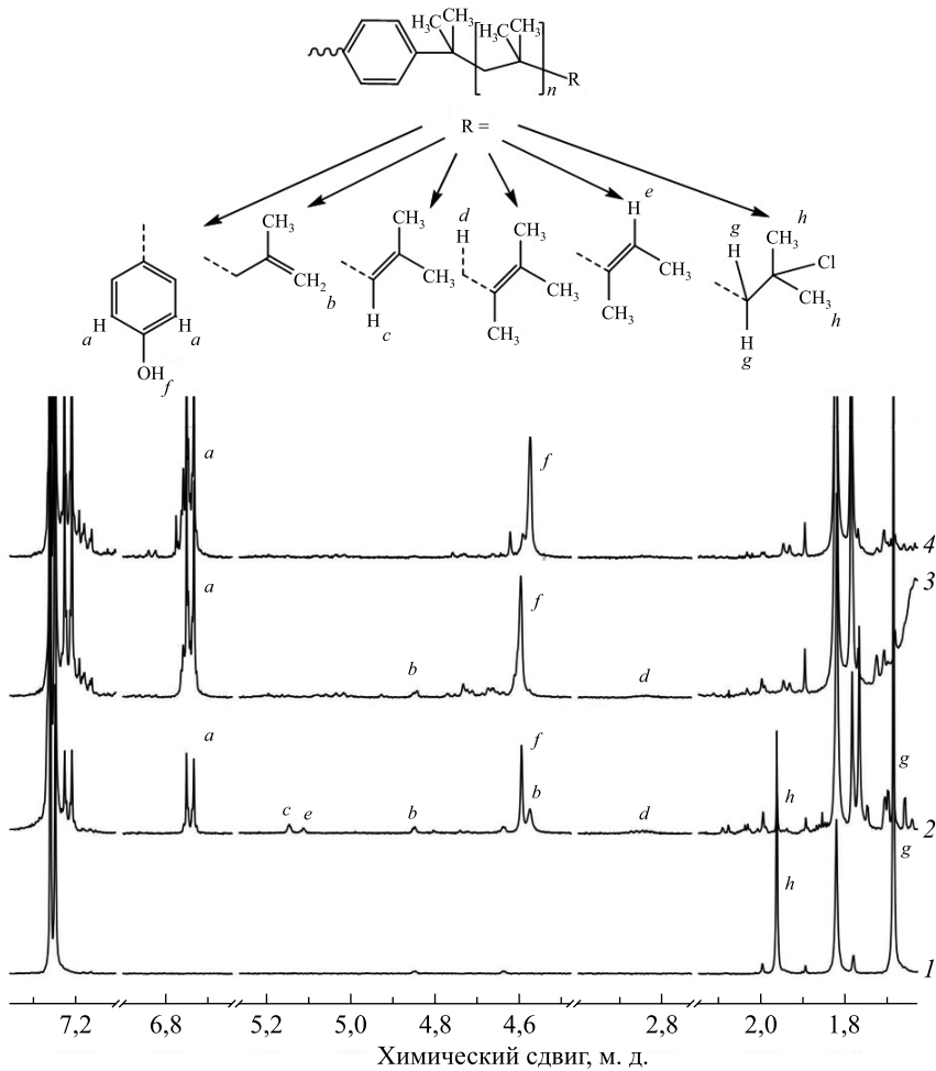
Рис. 4. Фрагменты спектров ЯМР ^1\text{H} ПИБ-ОН с различной степенью алкилирования (1 – 0 %, 2 – 36 %, 3 – 58 %, 4 – 89 %)
