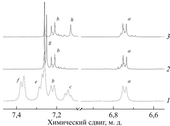
Рис. 6. Фрагменты спектров ЯМР ^1\text{H} ПИБ-ОН различной функциональности (1 – монофункциональный, 2 – дифункциональный, 3 – трифункциональный)
