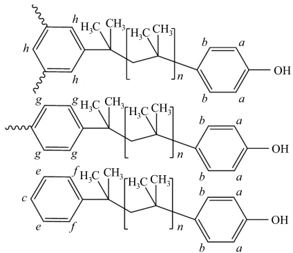
Рис. 6. Фрагменты спектров ЯМР ^1\text{H} ПИБ-ОН различной функциональности (1 – монофункциональный, 2 – дифункциональный, 3 – трифункциональный)
