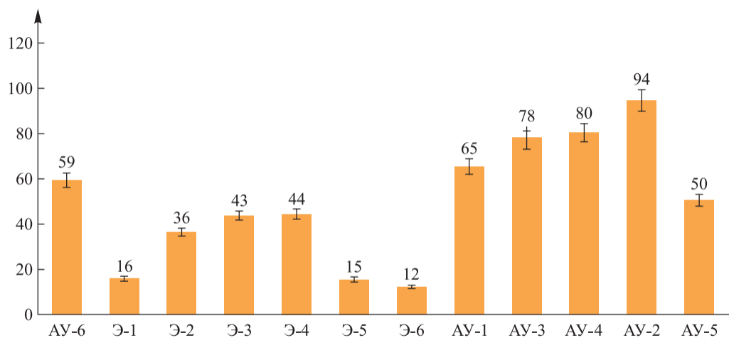
Рис. 2. Адсорбционная способность сорбентов по отношению к B_{12} , мг/г
