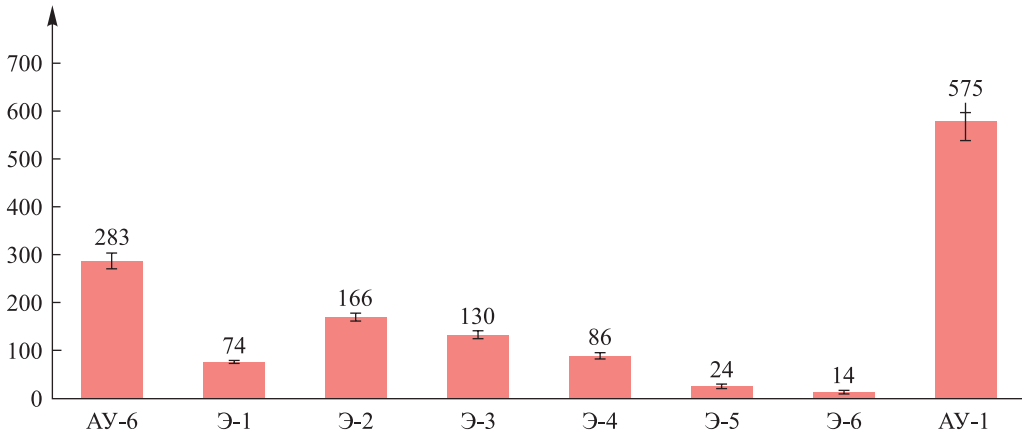
Рис. 3. Адсорбционная способность сорбентов по отношению к МО, мг/г
