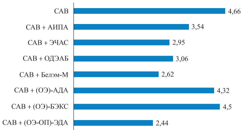
Рис. 3. Константы капиллярности для образцов САВ, c \cdot 10^{-8}, \text{cm}^5
