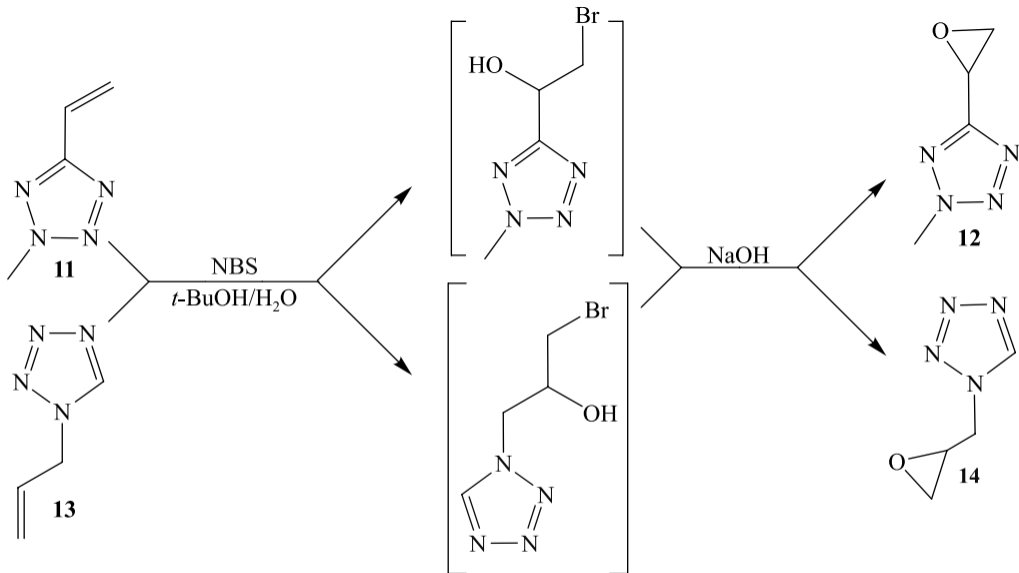
Рис. 5. Схема синтеза тетразолсодержащих эпоксидов 12 и 14
