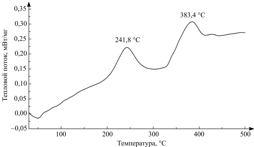
Рис. 1. Кривая дифференциальной сканирующей калориметрии для покрытия Ni–P
