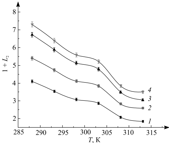
Рис. 3. Зависимость общего количества адсорбционных слоев молекул ЦЕФОТ ( 1 + L_2 ) от температуры ( T ):
