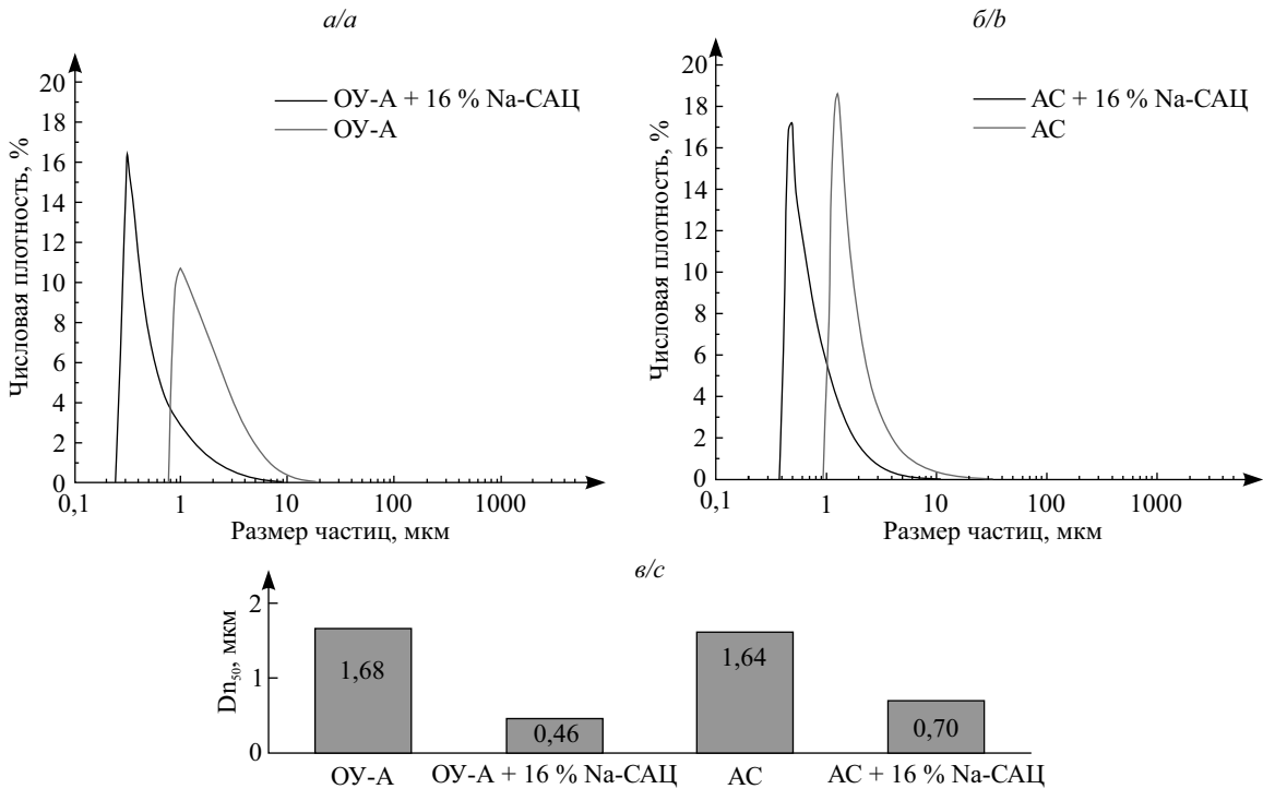
Рис. 6. Числовое распределение ( a , б ) и диаграмма медианных значений Dn_{50} ( в ) размеров частиц исходных и модифицированных АУ
