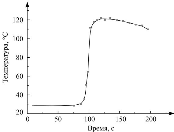
Рис. 1. Температурный профиль ФП АА с АNa в 1 % водном растворе ПАА.
