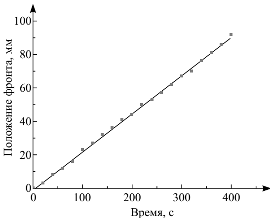
Рис. 2. Зависимость пройденного фронтом расстояния от времени при ФП АА с АNa в 1 % водном растворе ПАА.
