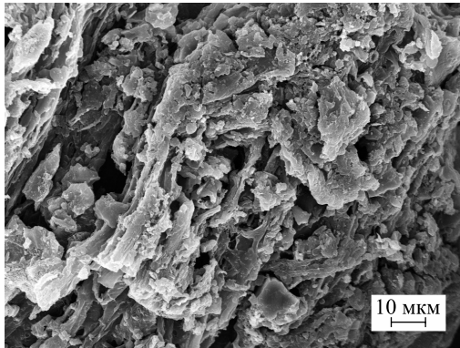
Рис. 10. СЭМ-фотографии АУ, полученного на основе ГЛ с использованием ДТ (а) и ИМ (б) в качестве активатора
