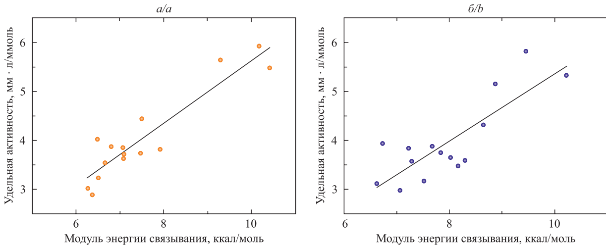
Рис. 9. Корреляция модуля энергии связывания и удельной активности соединений 1–5, 8–17 по отношению к E. coli ATCC 25922 (a) и S. aureus ATCC 6538 (б)
